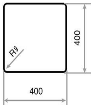
Отвор долно вграждане
